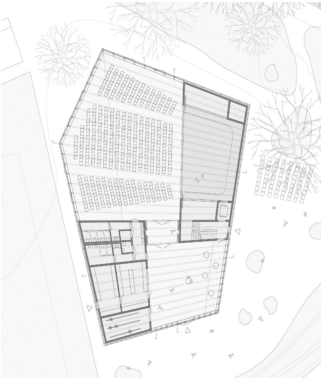
Grundriss Erdgeschoss
