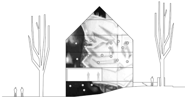
Ansicht Ostfassade
